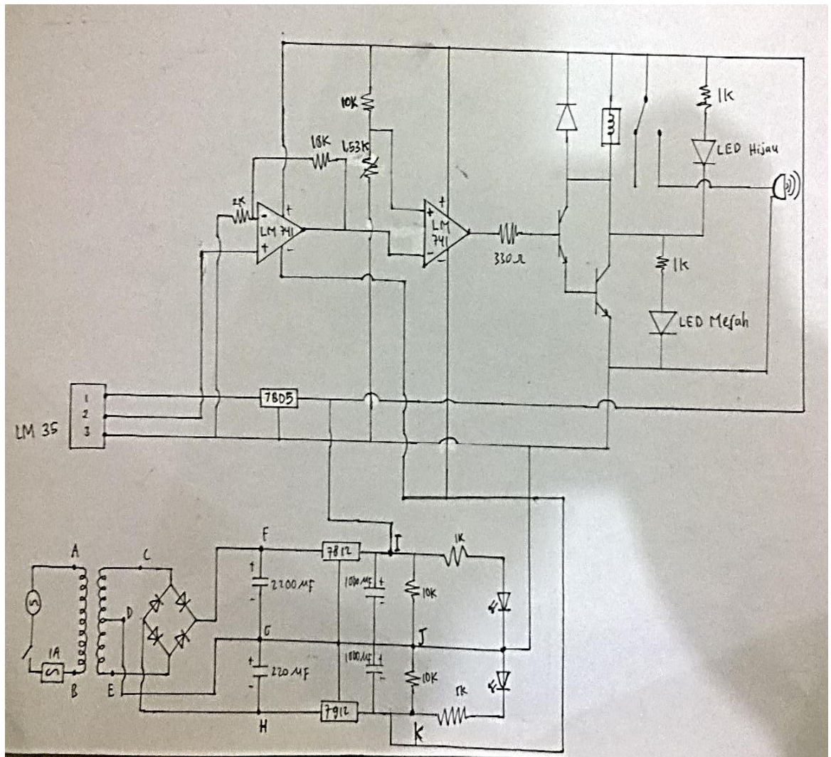
Gambar Rangkaian sensor suhu dengan IC LM35
